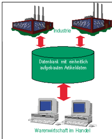
Funktionsschema Artikelstammdatenbank
